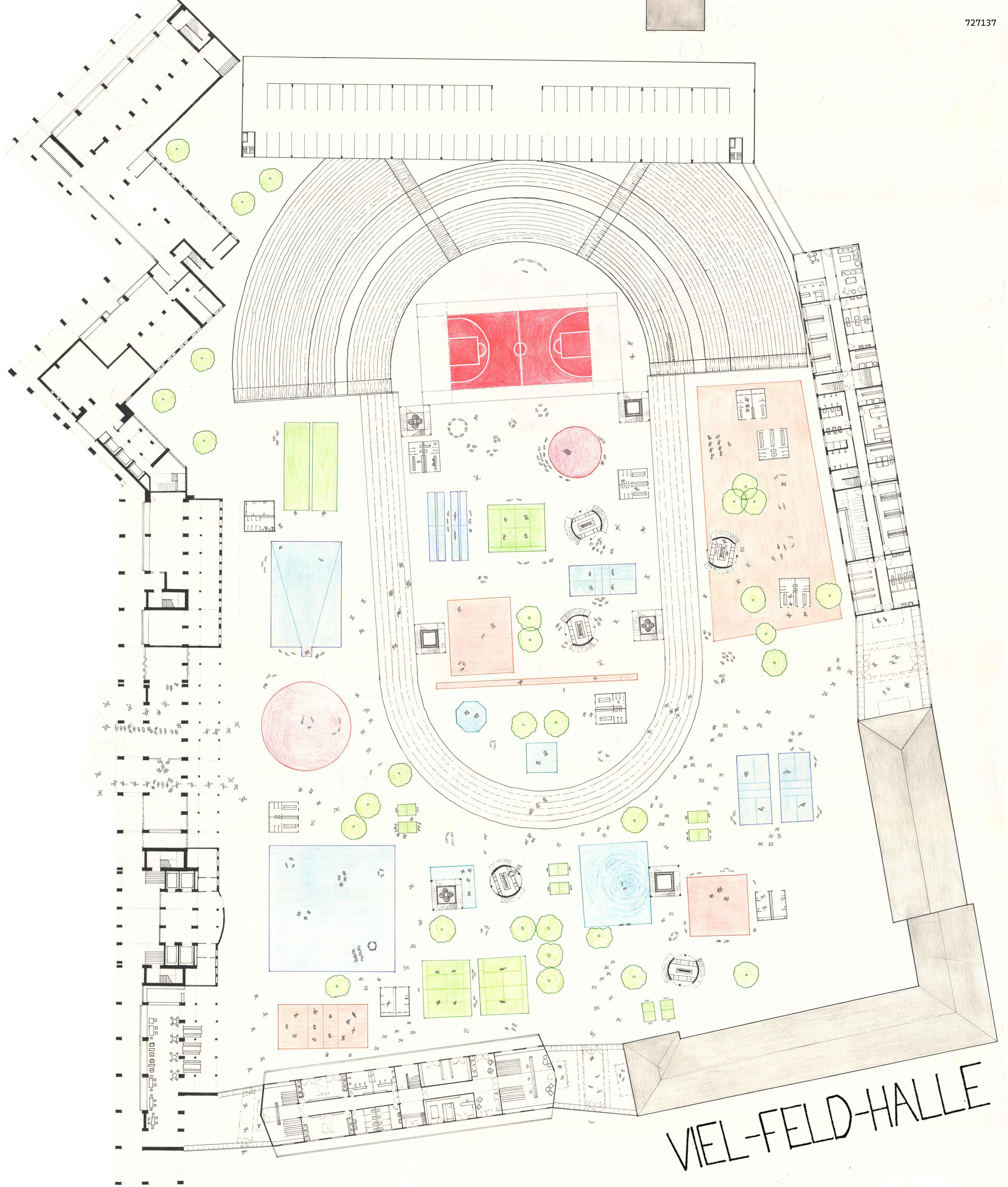
Grundriss 1:250
