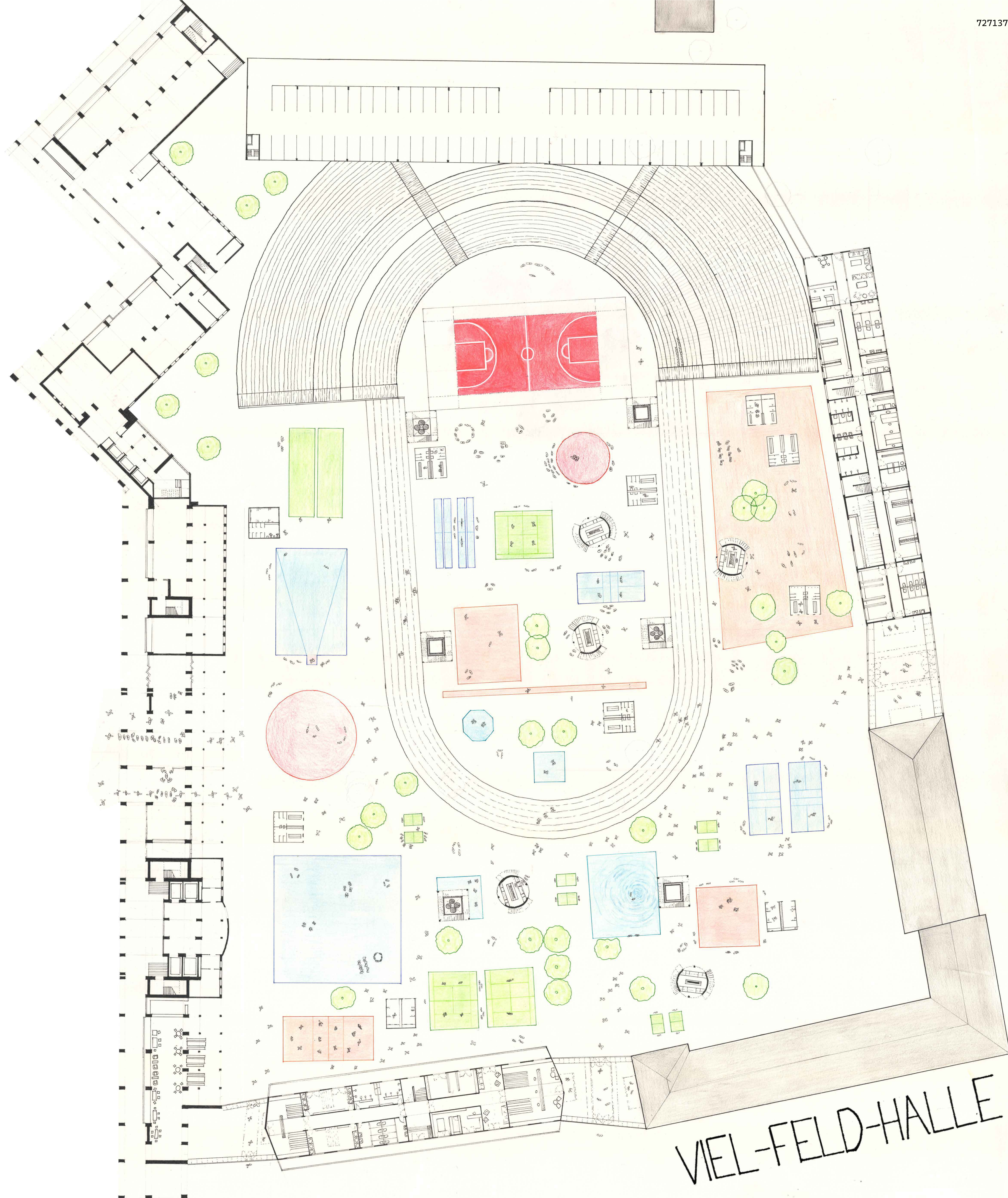
Grundriss 1:250
