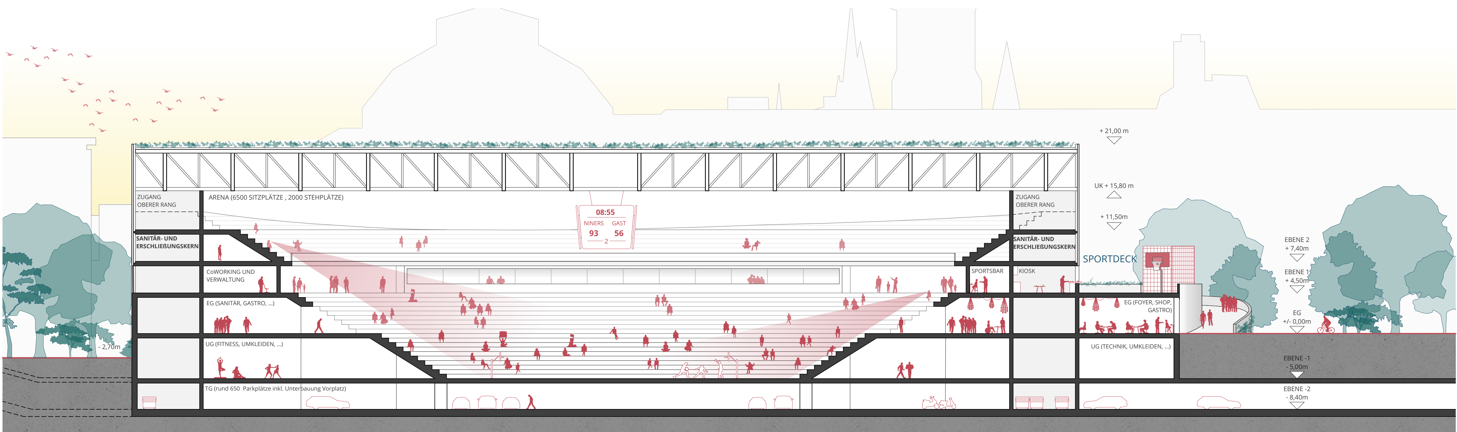
LÄNGSSCHNITT M1:250
