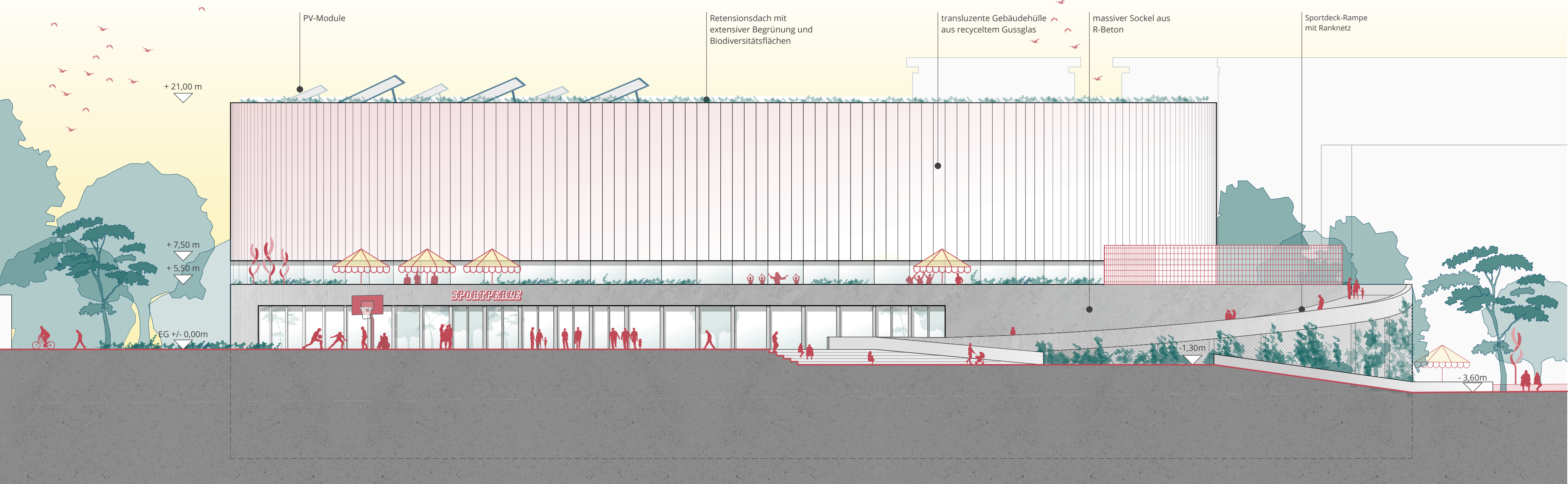
OSTANSICHT M1:250
