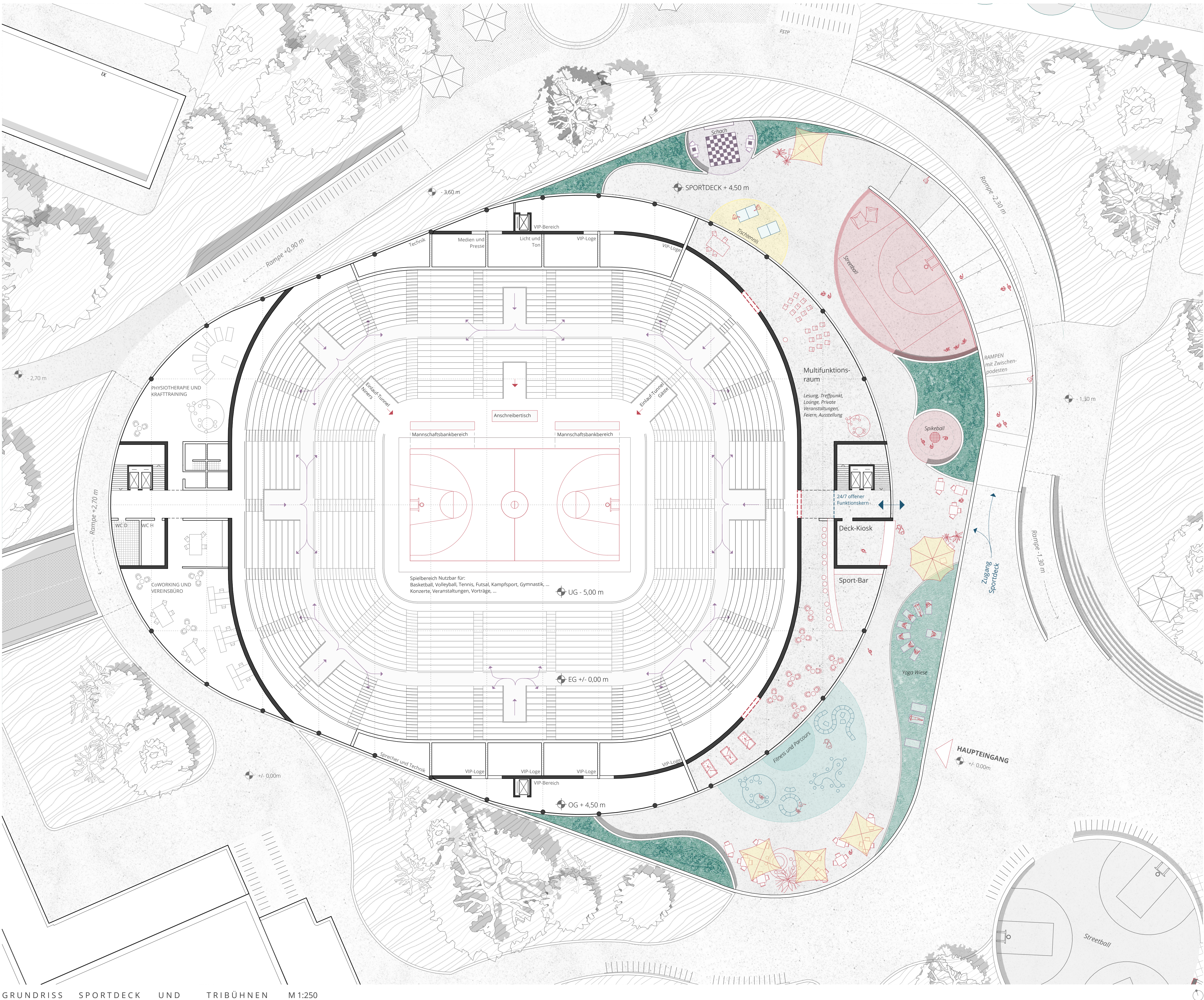
GRUNDRISS SPORTDECK UND TRIBÜHNEN M1:250
