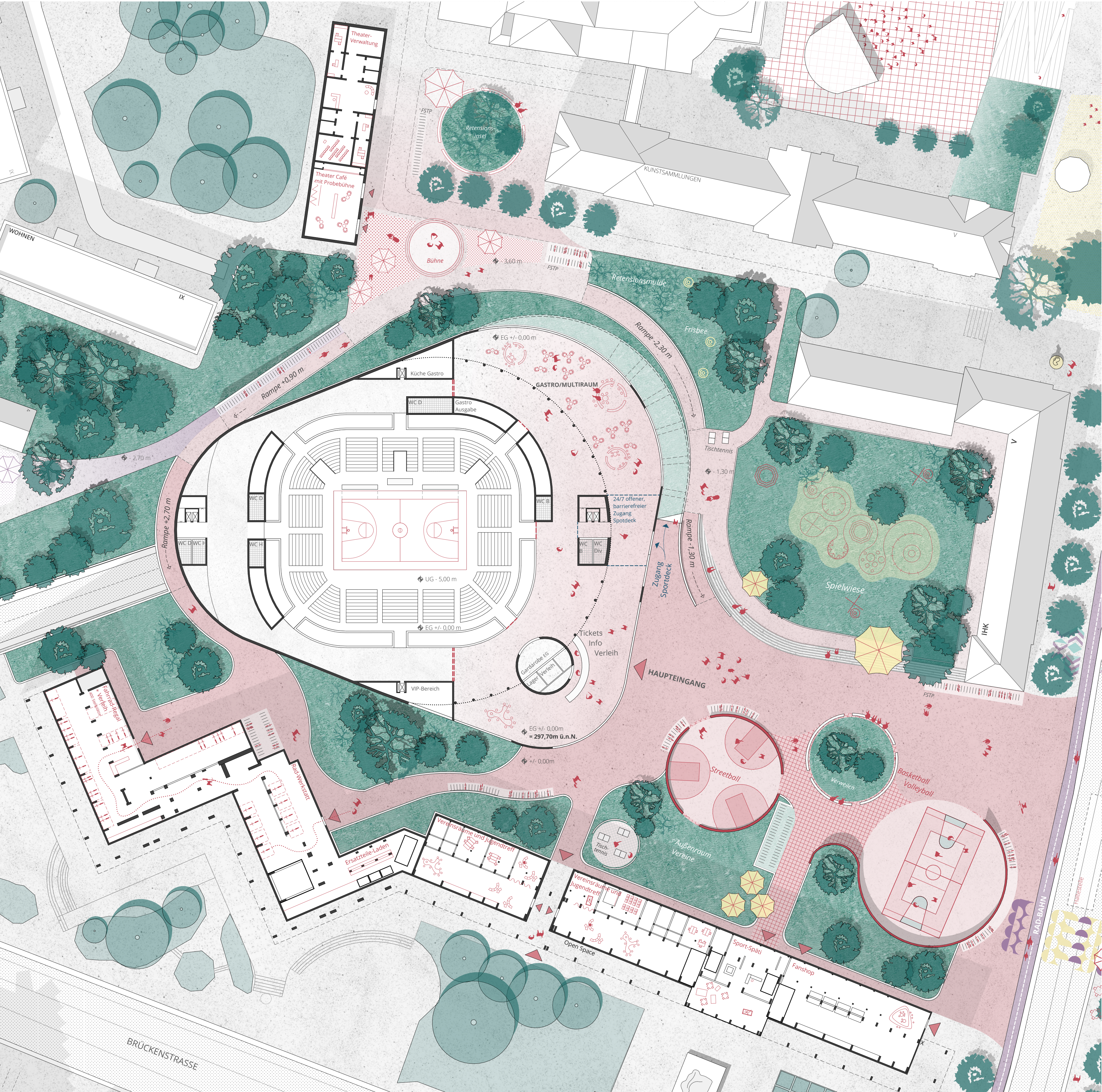
LAGEPLAN UND ERDGESCHOSSGRUNDRISS M1:500
