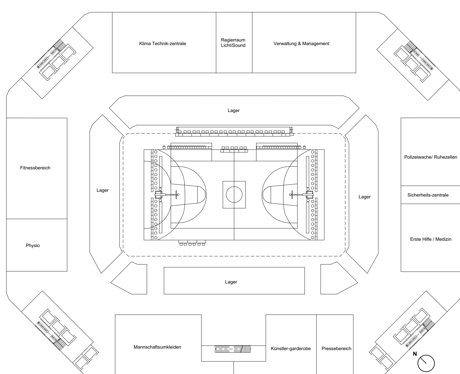
Grundriss UG M 1:500
