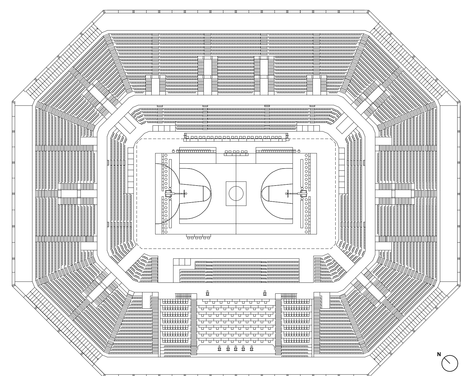
Tribünensitzplan M 1:500
