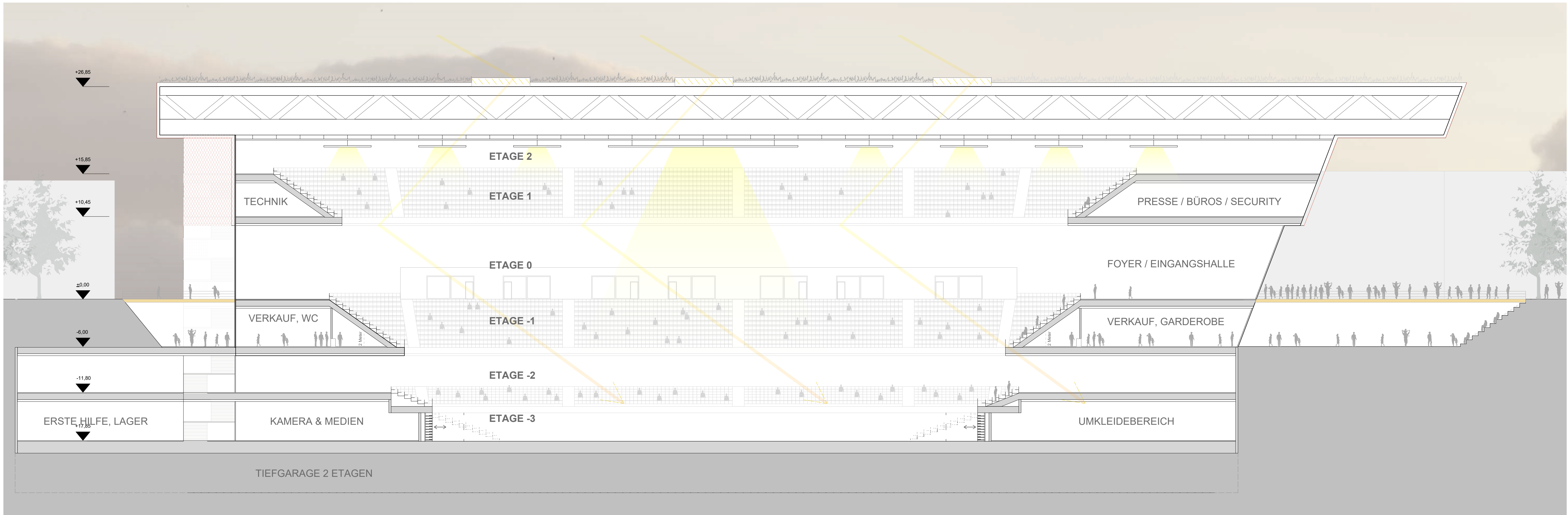
SCHNITT M 1:250
