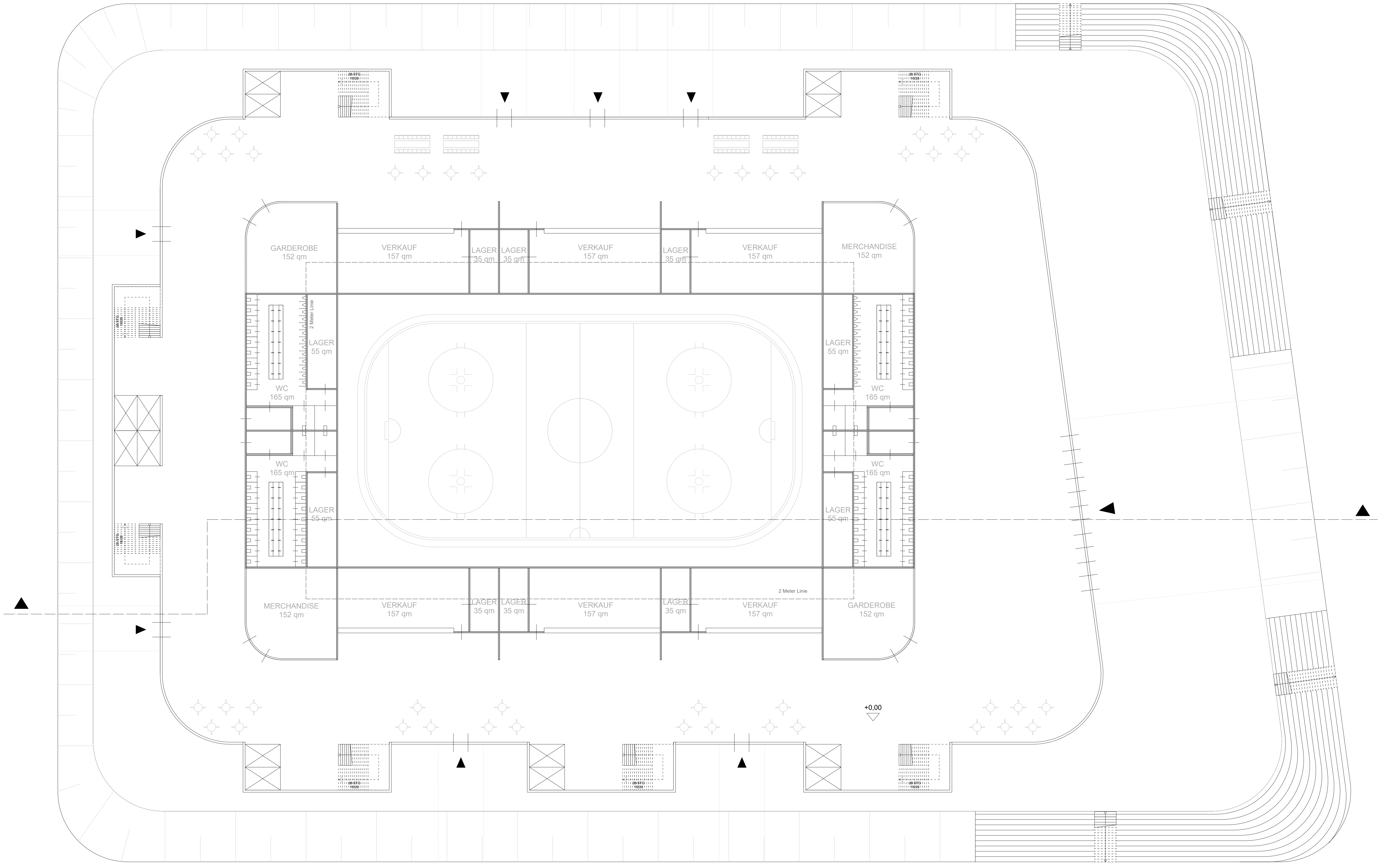
GRUNDRISS EBENE -1 M 1:250
